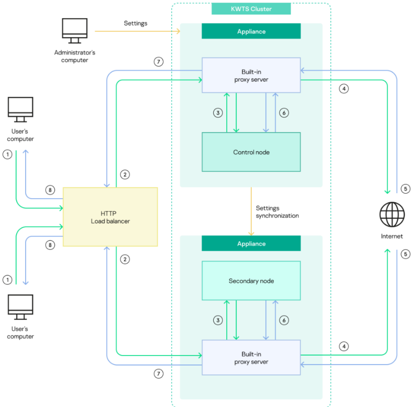
Рисунок 5. Схема подключения балансировщика при использовании встроенного прокси-сервера
