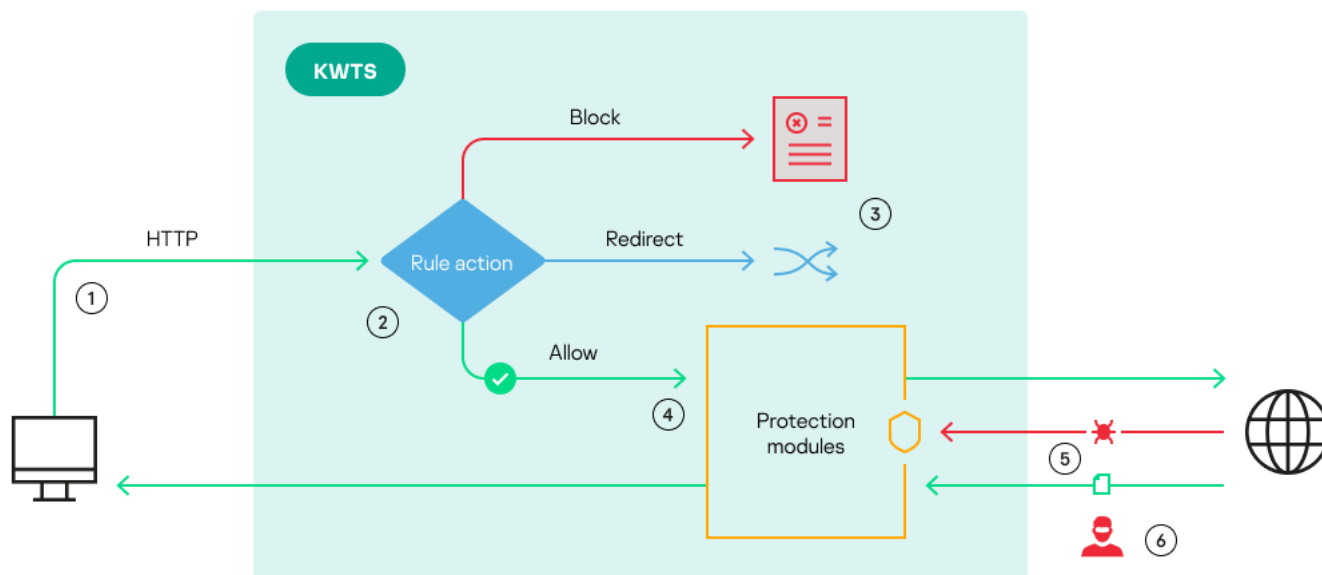
Рисунок 7. Принципы обработки HTTP-сообщений
