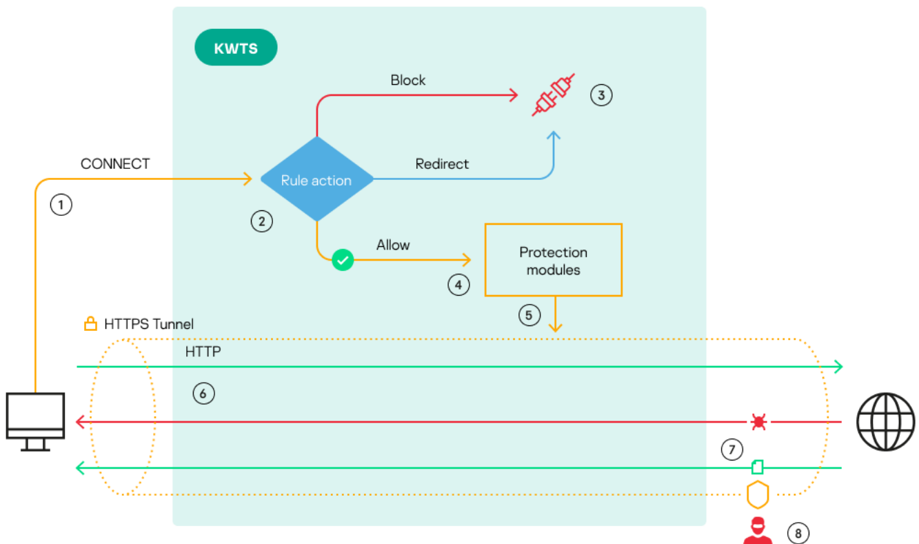
Рисунок 8. Механизм обработки зашифрованных соединений по умолчанию
