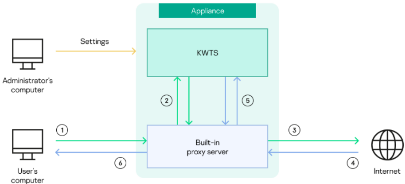
Рисунок 1. Принцип работы приложения Kaspersky Web Traffic Security
