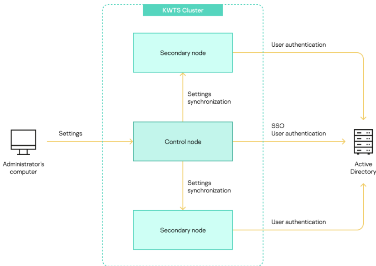
Рисунок 3. Схема взаимодействия компонентов приложения
